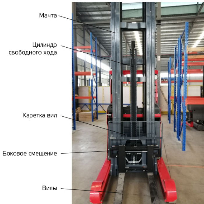
Рисунок 7. Основные элементы ричтрака. Вид спереди
