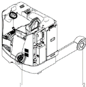
Рисунок 37. Проверка колес
