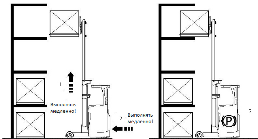
Рисунок 29. Подъем груза
