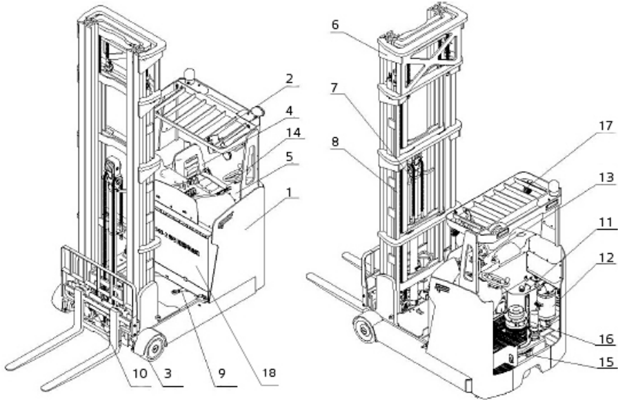
Рисунок 4. Основная конструкция электрического ричтрака
