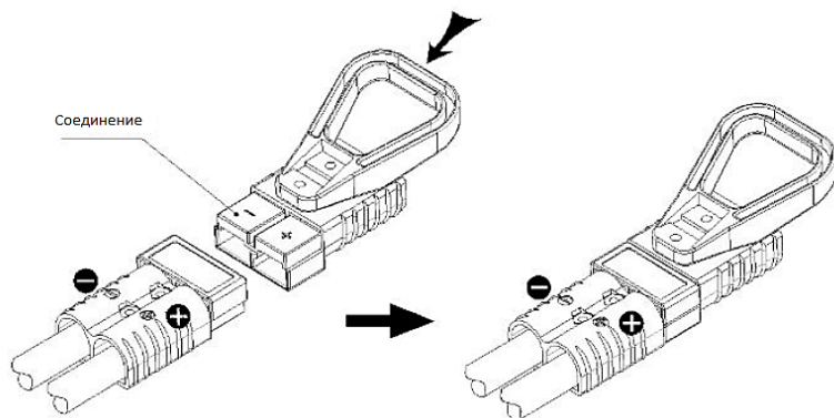
Рисунок 23. Подключение аккумулятора
