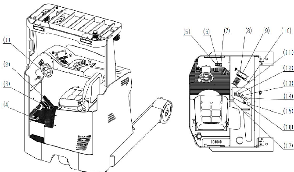
Рисунок 9. Положение рычагов управления и приводного механизма
