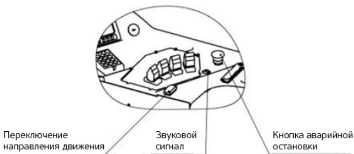
Рисунок 19. Основные кнопки
