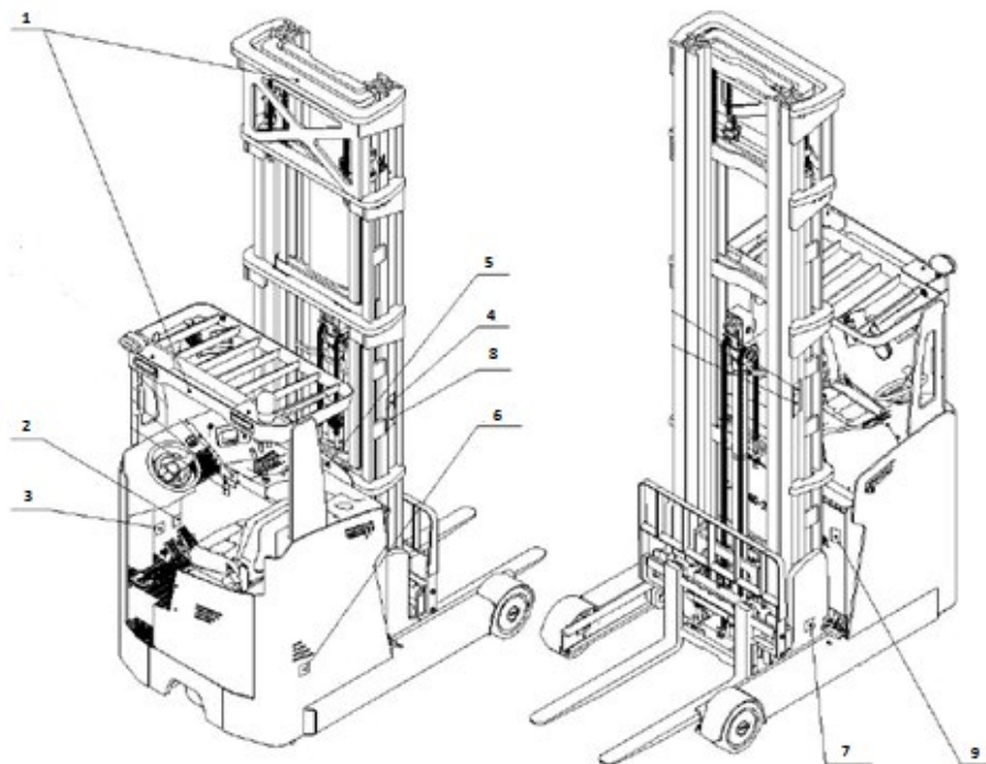
Рисунок 22. Расположение основных наклеек
