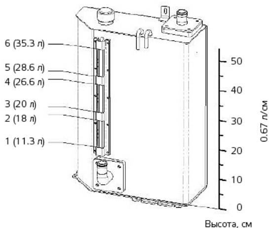
Рисунок 39. Объем масляного бака
