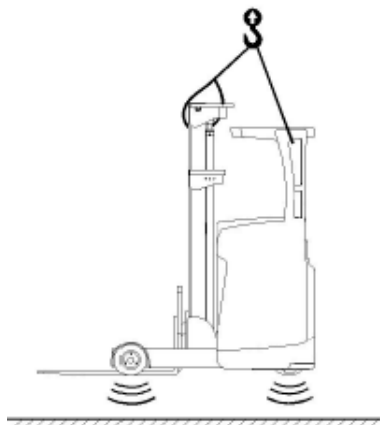
Рисунок 33. Крепление ричтрака при подъеме
