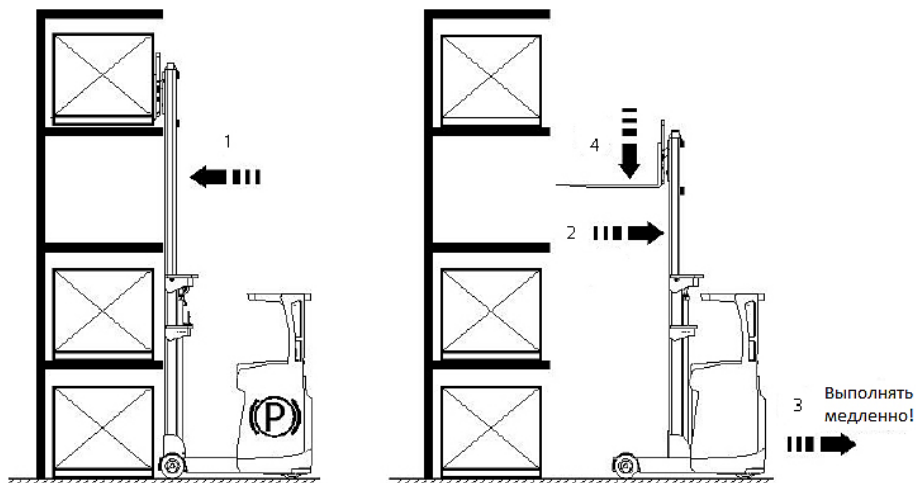
Рисунок 30. Укладка груза
