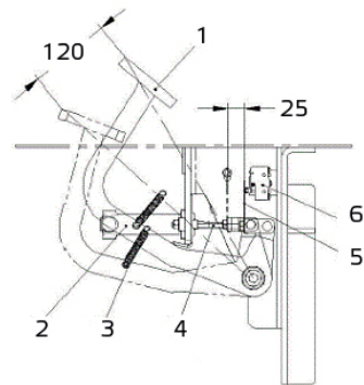
Рисунок 17. Строение педали тормоза
