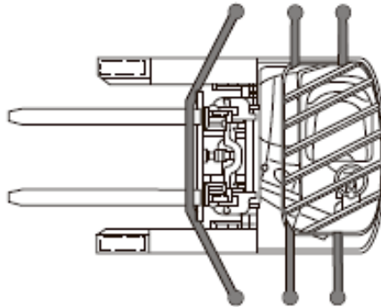
Рисунок 32. Закрепления ричтрака при транспортировке. Вид сверху
