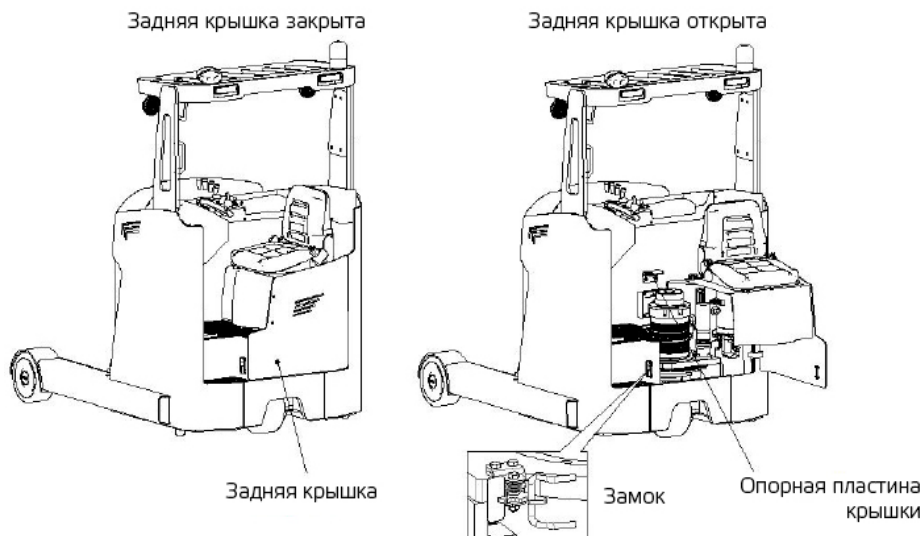
Рисунок 8. Положение задней крышки ричтрака
