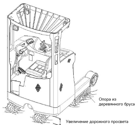
Рисунок 34. Положение ричтрака во время длительного хранения
