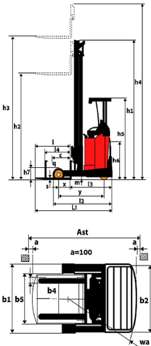
Рисунок 1. Технические характеристики ричтрака
