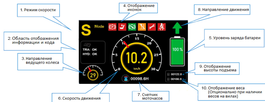
Рисунок 36. Индикатор заряда батареи на дисплее ричтрака
