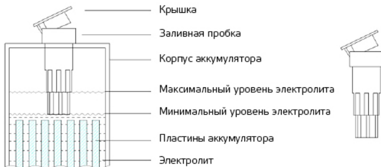
Рисунок 35. Проверка уровня электролита в аккумуляторе ричтрака
