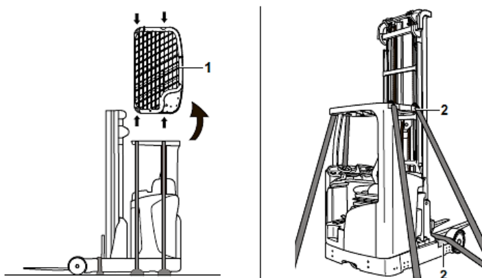
Рисунок 31. Закрепление ричтрака для транспортировки
