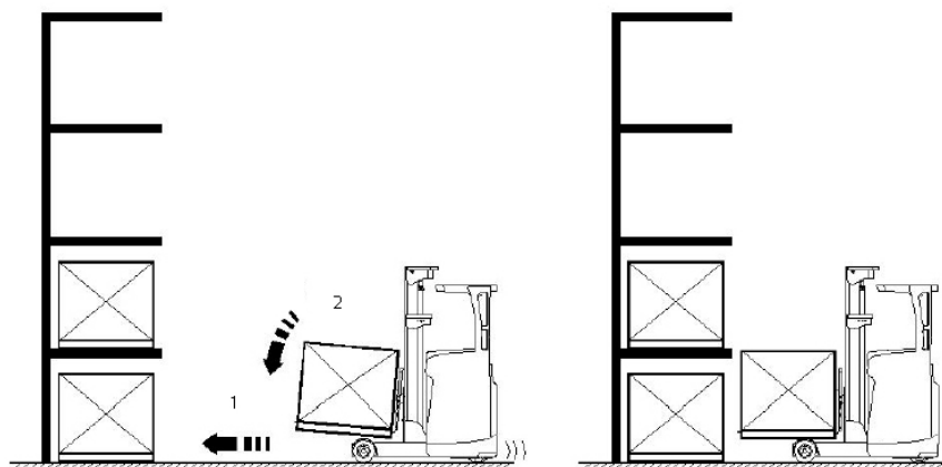
Рисунок 28. Транспортировка груза к месту хранения
