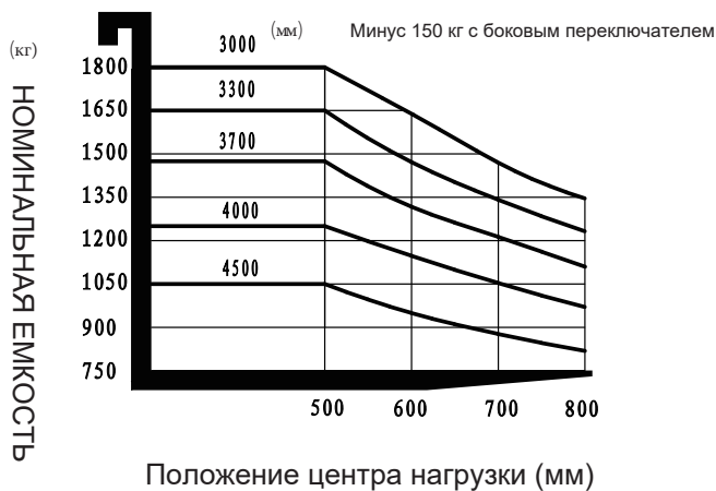
ГРАФИК НОМИНАЛЬНЫХ МОЩНОСТЕЙ И ЦЕНТРОВ НАГРУЗКИ
